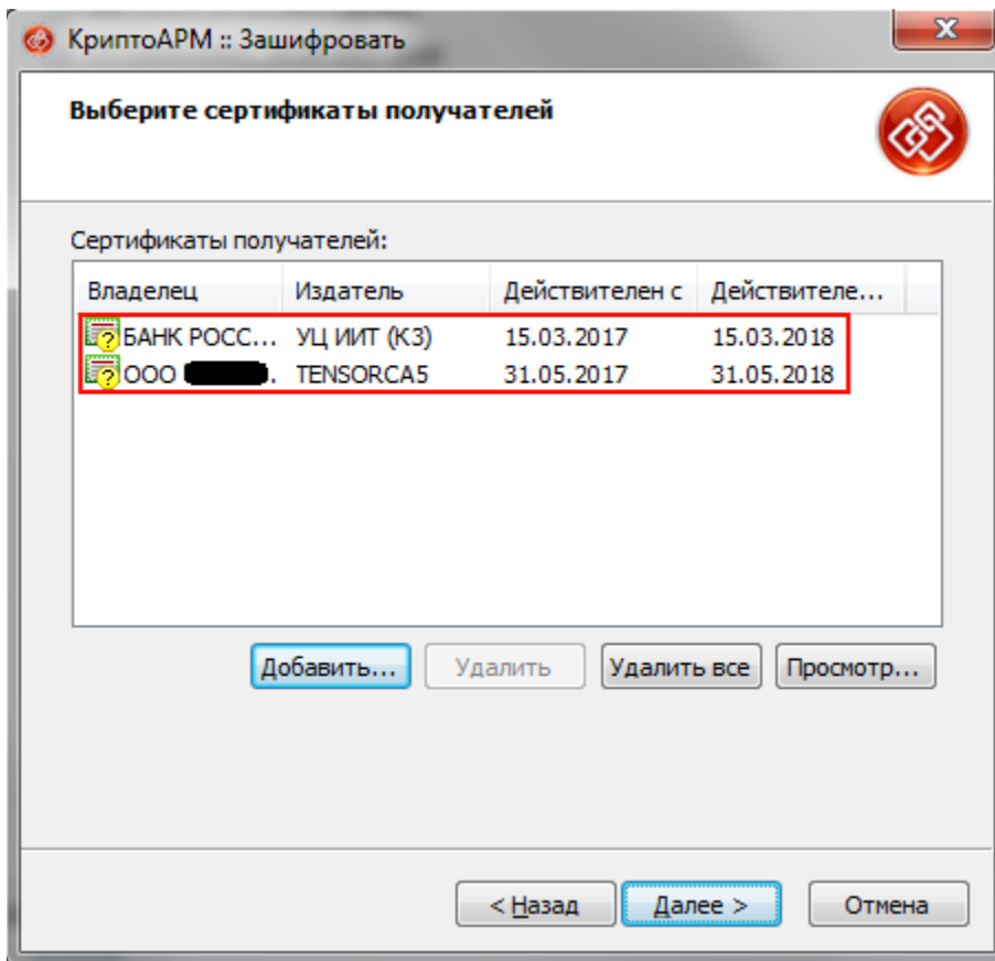
Рисунок 9 - Выбор сертификатов
