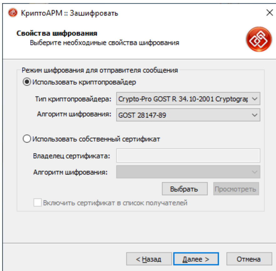
Рисунок 8 - Выбор криптопровайдера
