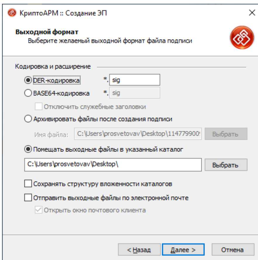
Рисунок 7 – Выбор кодировки
