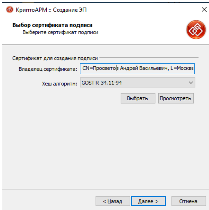
Рисунок 4 – Выбор УКЭП
