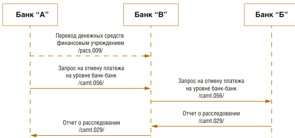
Рисунок 16. Обмен сообщениями, сценарий 2 10
