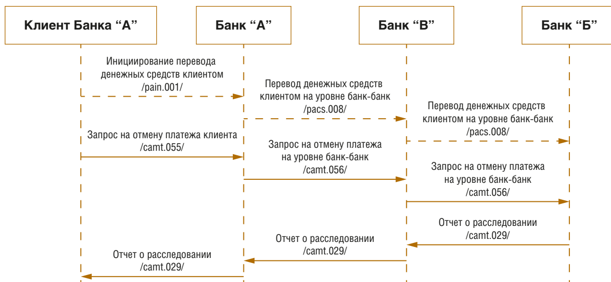
Рисунок 15. Обмен сообщениями, сценарий 1 9
