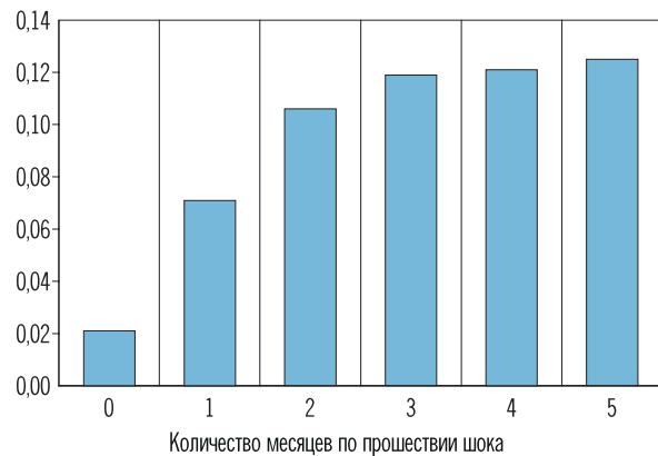
Кумулятивный отклик потребительской инфляции на 1%-ное изменение номинального эффективного курса рубля к иностранным валютам (расчеты по VAR-модели, процентных пунктов)
