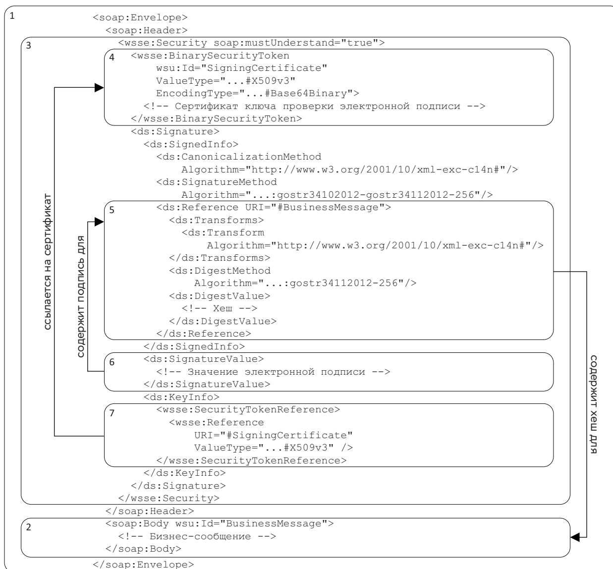
РИСУНОК А.1. СХЕМА ПОДПИСАНИЯ СООБЩЕНИЯ
