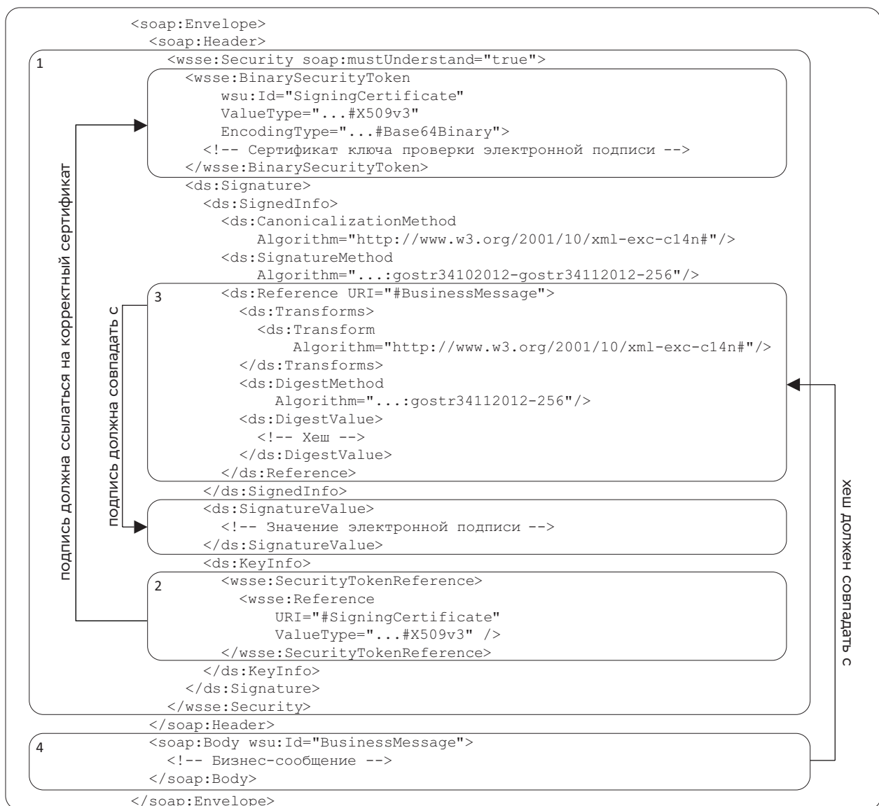
РИСУНОК А.2. СХЕМА ПРОВЕРКИ ЭЛЕКТРОННОЙ ПОДПИСИ
