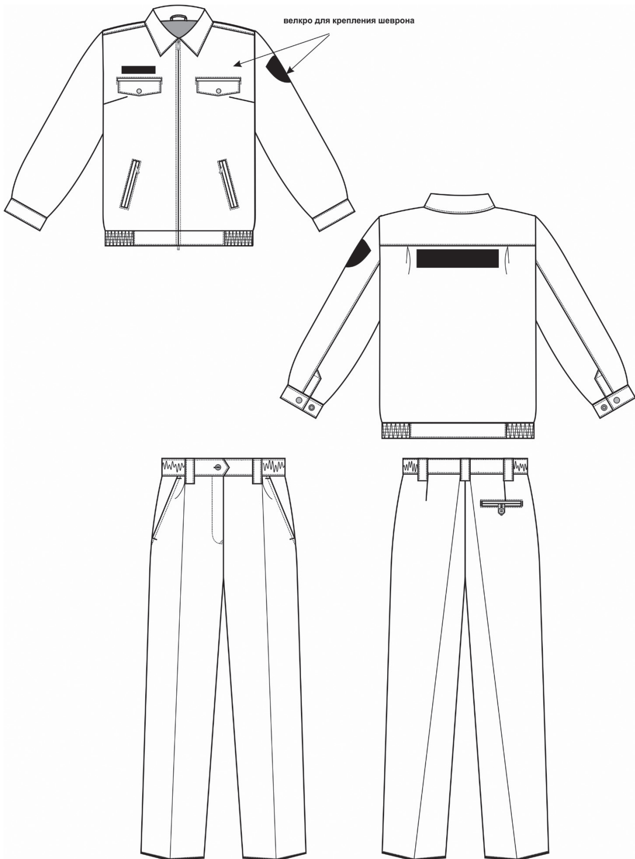
РИСУНОК 10. КОСТЮМ ЖЕНСКИЙ ДЛЯ ЗАЩИТЫ ОТ ОБЩИХ ПРОИЗВОДСТВЕННЫХ ЗАГРЯЗНЕНИЙ И МЕХАНИЧЕСКИХ ВОЗДЕЙСТВИЙ
