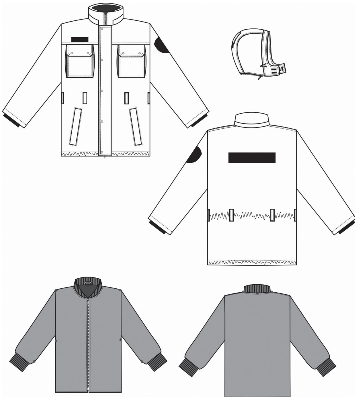
РИСУНОК 6. КУРТКА МУЖСКАЯ ДЛЯ ЗАЩИТЫ ОТ ПОНИЖЕННЫХ ТЕМПЕРАТУР
